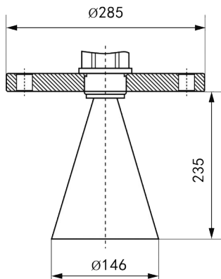
DN150
