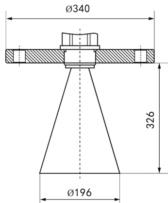
DN200
